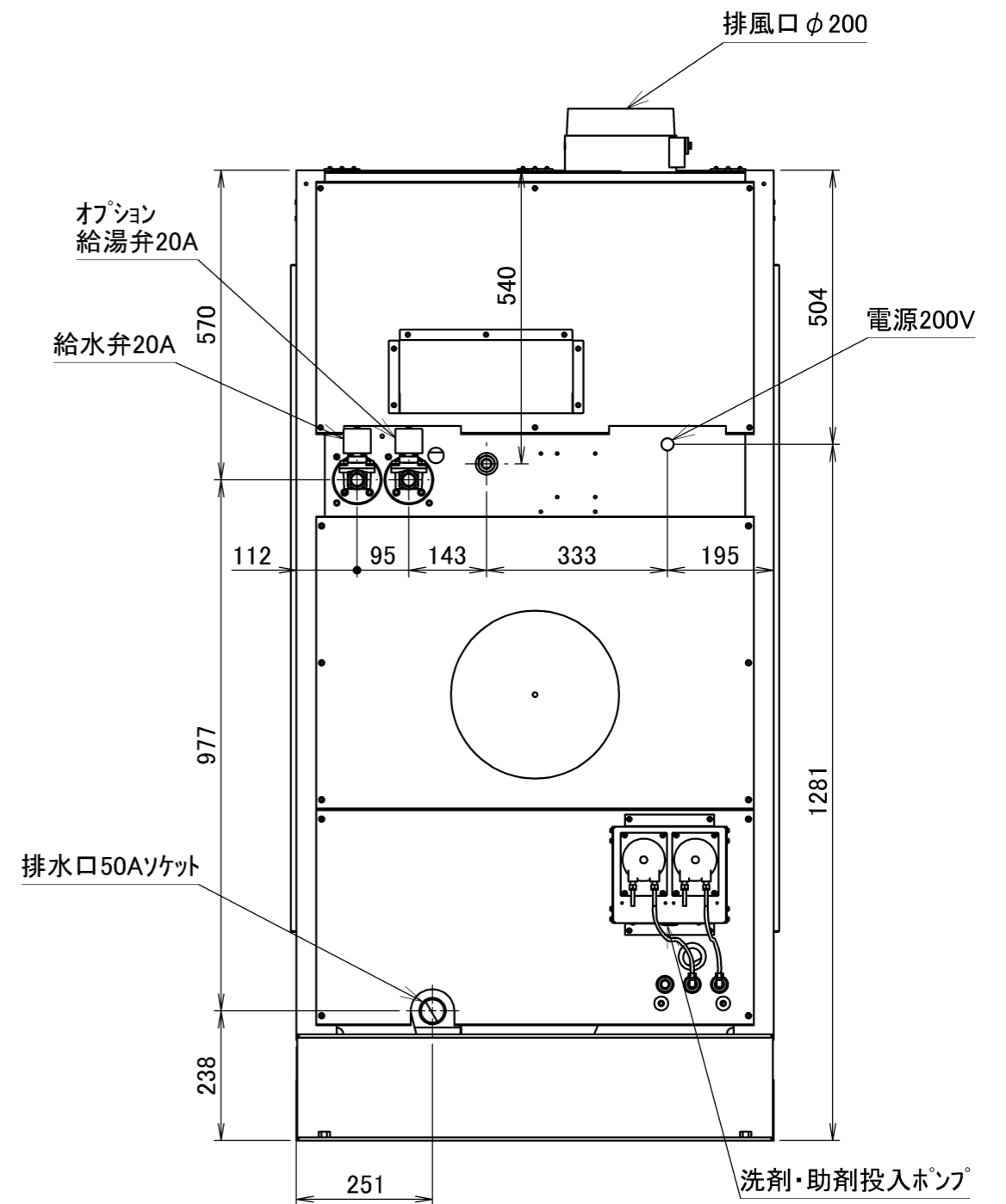
コイン洗濯乾燥機 WD171CS 外観図
